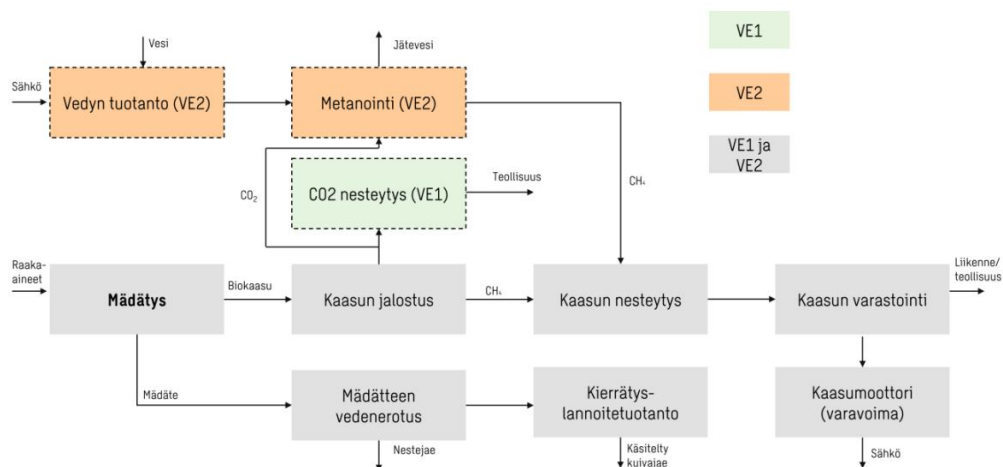
Kuva 2-2. Laitoksen alustavat pääprosessit ja -virrat.
